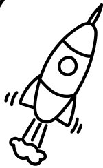
MARS
