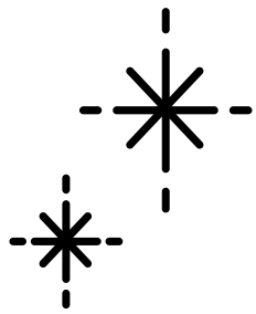
MARS
