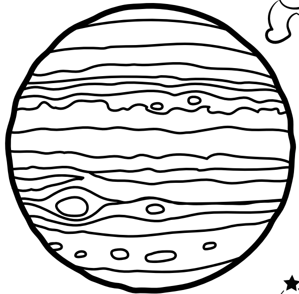
JUPITER
